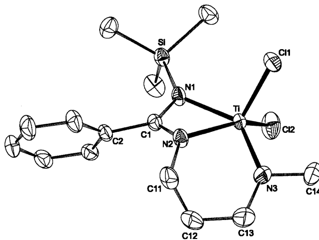
Figure 1. Molecular structure of compound 3 ; thermal ellipsoids are drawn at the 50% probability level; \text{Ti}-\text{Cl}(1) 2.2464(6), \text{Ti}-\text{Cl}(2) 2.2954(7), \text{Ti}-\text{N}(1) 2.077(2), \text{Ti}-\text{N}(2) 2.059(2), \text{Ti}-\text{N}(3) 1.863(2) Å; \text{Cl}(1)-\text{Ti}-\text{Cl}(2) 107.26(2), \text{N}(1)-\text{Ti}-\text{N}(2) 64.03(6), \text{N}(1)-\text{Ti}-\text{N}(3) 139.40(7), \text{N}(2)-\text{Ti}-\text{N}(3) 84.08(7), \text{N}(3)-\text{Ti}-\text{Cl}(1) 107.72(6), \text{N}(3)-\text{Ti}-\text{Cl}(2) 100.83(6), \text{Ti}-\text{N}(3)-\text{C}(13) 137.0(2), \text{Ti}-\text{N}(3)-\text{C}(14) 110.2(2) ^\circ .
